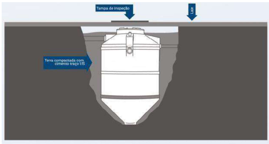
IMAGEM 02: Ilustração das etapas de escavação, compactação e laje.
