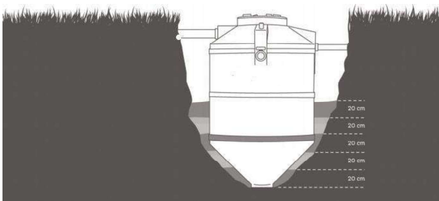
IMAGEM 01: Ilustração das etapas de escavação e compactação.
