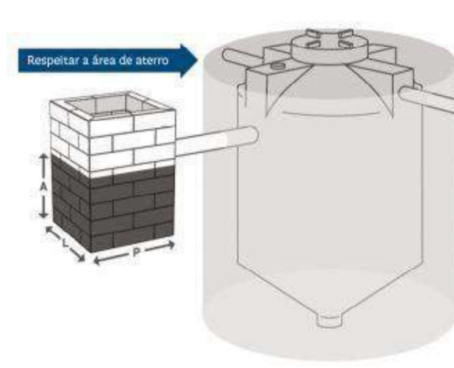
IMAGEM 03: Ilustração da caixa de secagem FONTE: Manual de Instalação Biodigestor 2022 - Acqualimp
